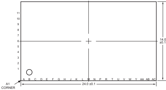
详细视图
