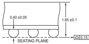
详细视图
